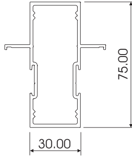
CLIP44 26 MULLION CL01A
