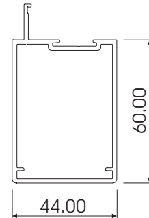
CLIP44 R11 DOOR JAMB CL218
