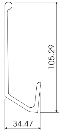
CLIP44 UNIVERSAL DOOR HANDLE CL37
